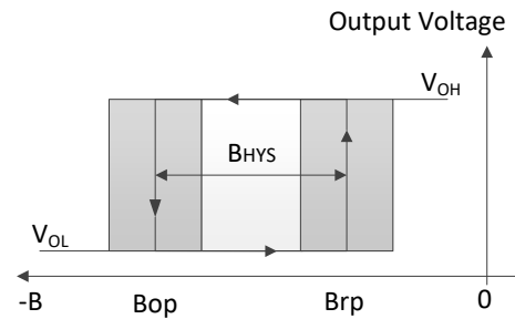
SOT23-3L output status
